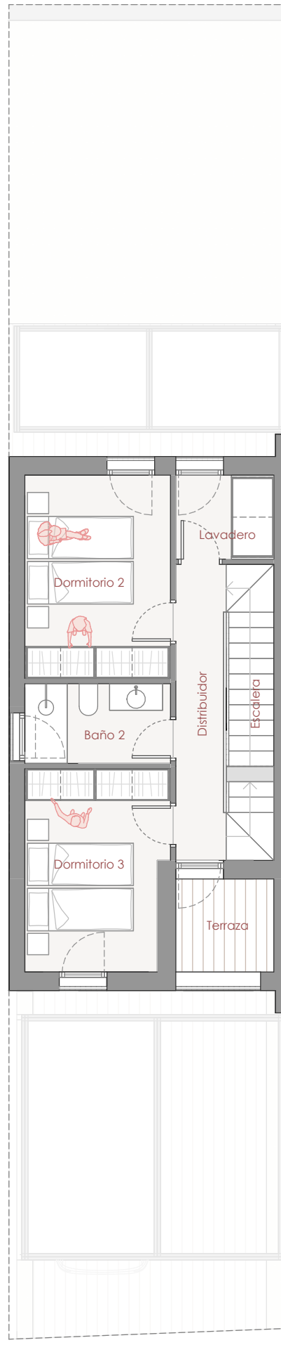
PLANTA PRIMERA
