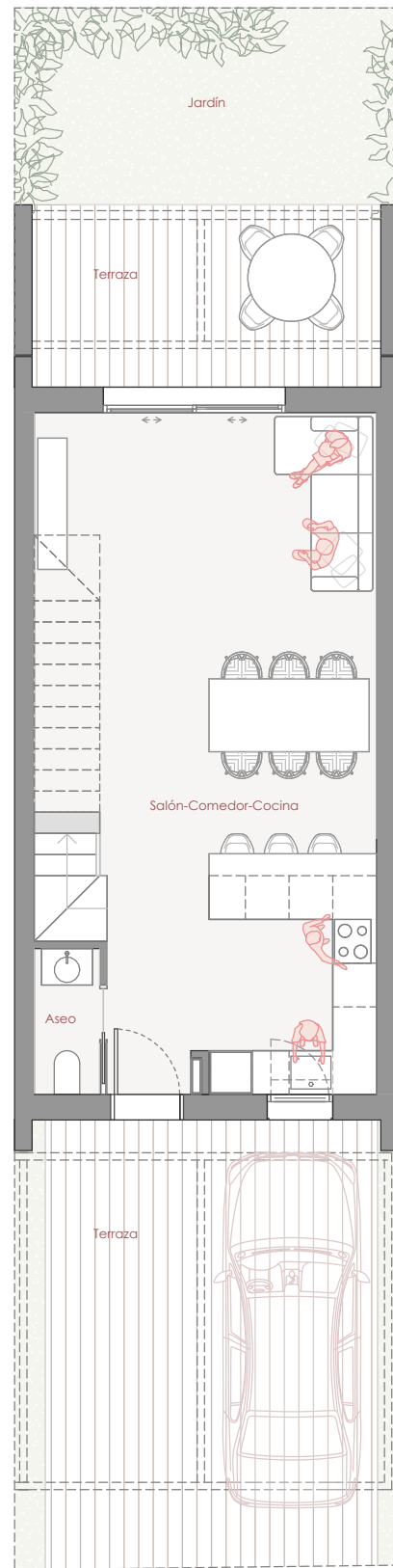
PLANTA BAJA
