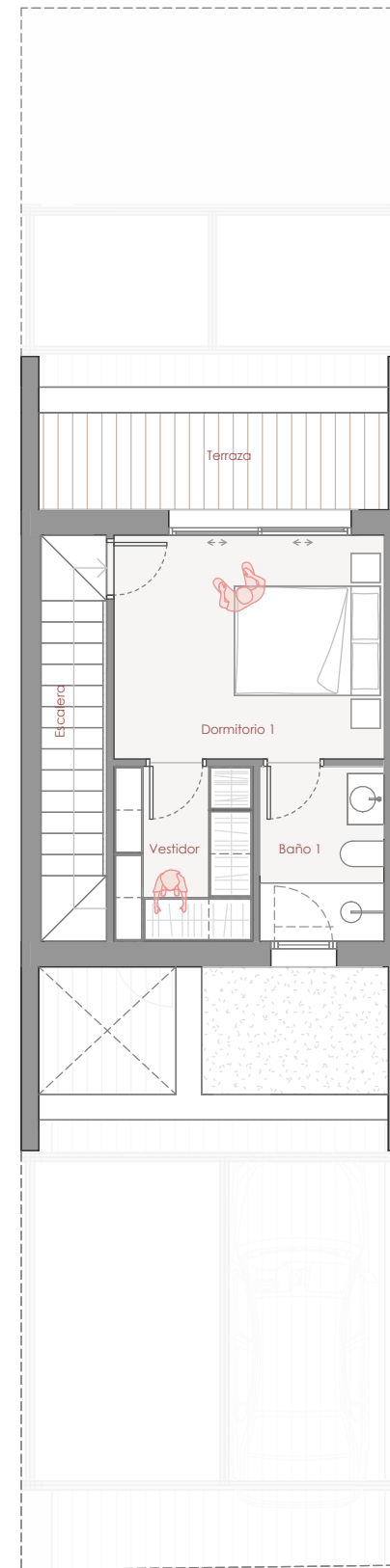
PLANTA SEGUNDA
