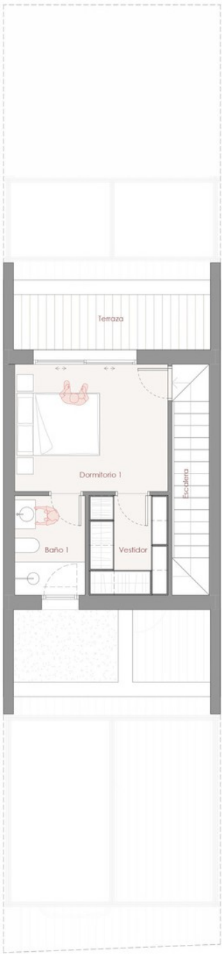
PLANTA SEGUNDA
