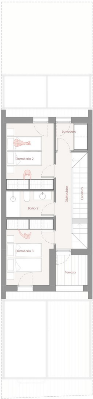
PLANTA PRIMERA
