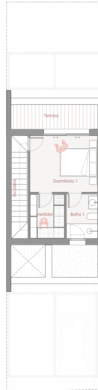
PLANTA SEGUNDA
