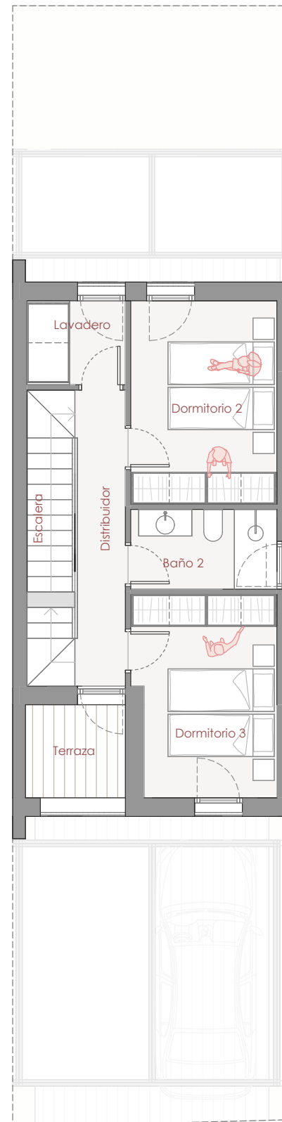
PLANTA PRIMERA
