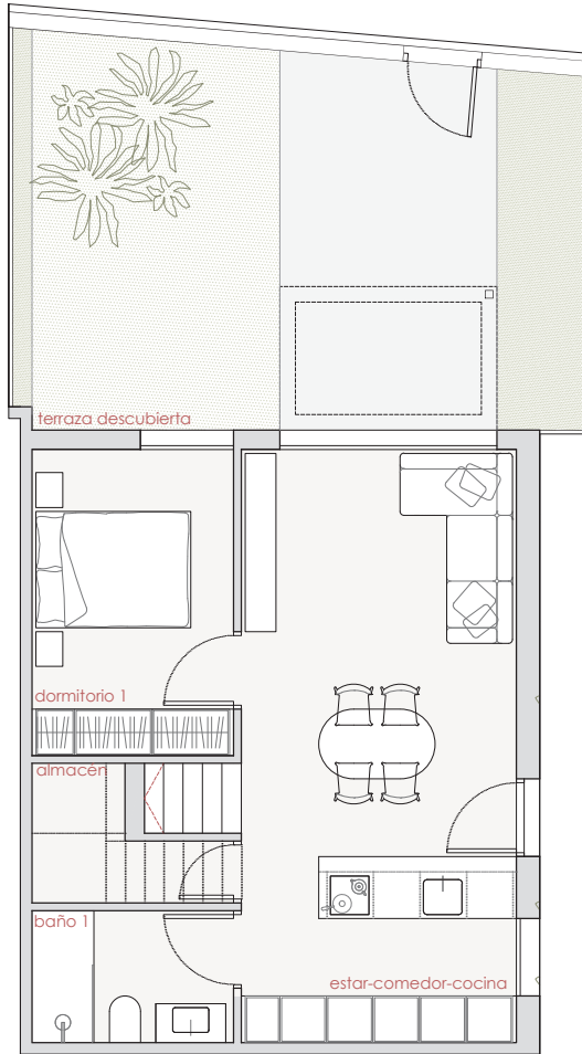
PLANTA BAJA + ZONA EXTERIORES
