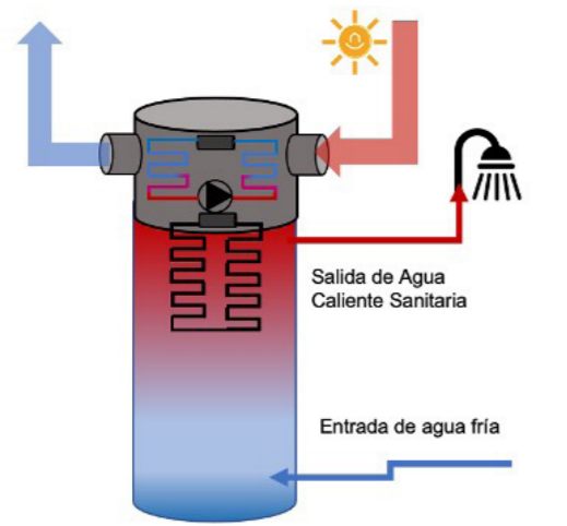
Kit compacto de aerotermia para ACS
